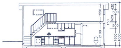
SEKTION A-A
