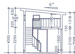
SEKTION B-B
